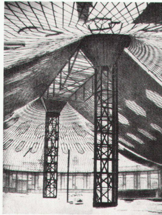
Vladimir Suchov: Pavillon der Industrie auf der Kunst- und Industrieausstellung, Nizhny-Novgorod (1898).
