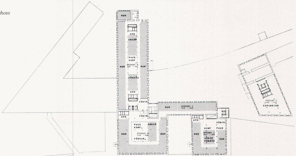
Grundriss Erdgeschoss
