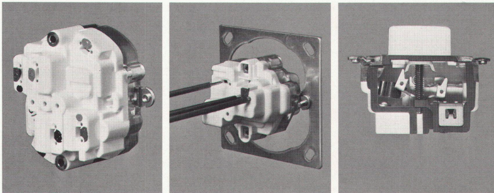
Gekapselter Sockel staubgeschützt und berührungssicher
