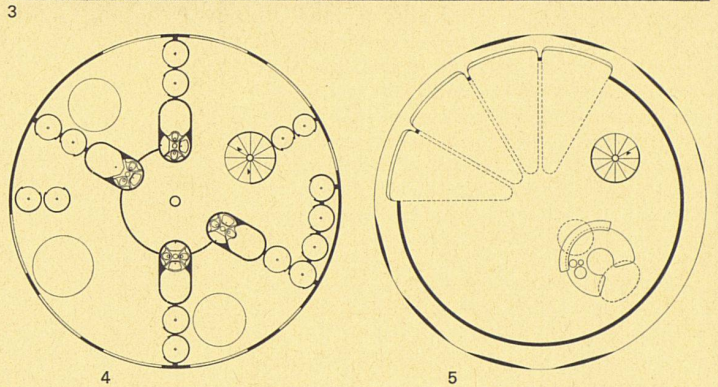
3-6 Kugelhaus Architekt: Roland R. Hanselmann, Olten Das Kugelhaus aus leichten Materialien ist drehbar auf einen Mast montiert und hat drei beliebig aufteilbare Geschosse. Die Einteilung erfolgt mittels zylindrischer Schrankelemente und Naßzellen
