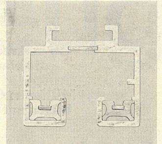
solide Leichtmetall-Stromschiene
