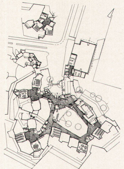
6-8 Grundschule in Berlin-Reinickendorf, Senftenberger Ring. Architekt: Dipl.-Ing. S. Heise 6 Grundriß Erdgeschoß
