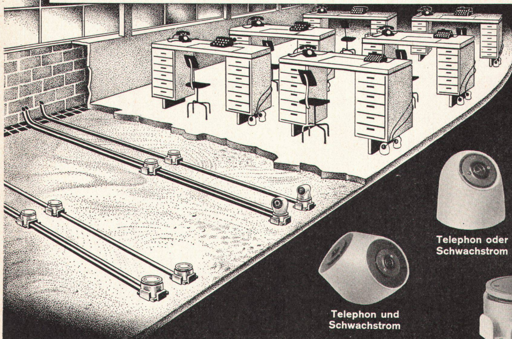
Bodendose mit Regulierung zur bodenbündigen Einstellung des Dosendeckels
