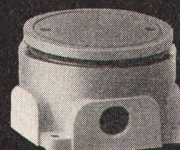
Bodendose mit Regulierung zur bodenbündigen Einstellung des Dosendeckels
