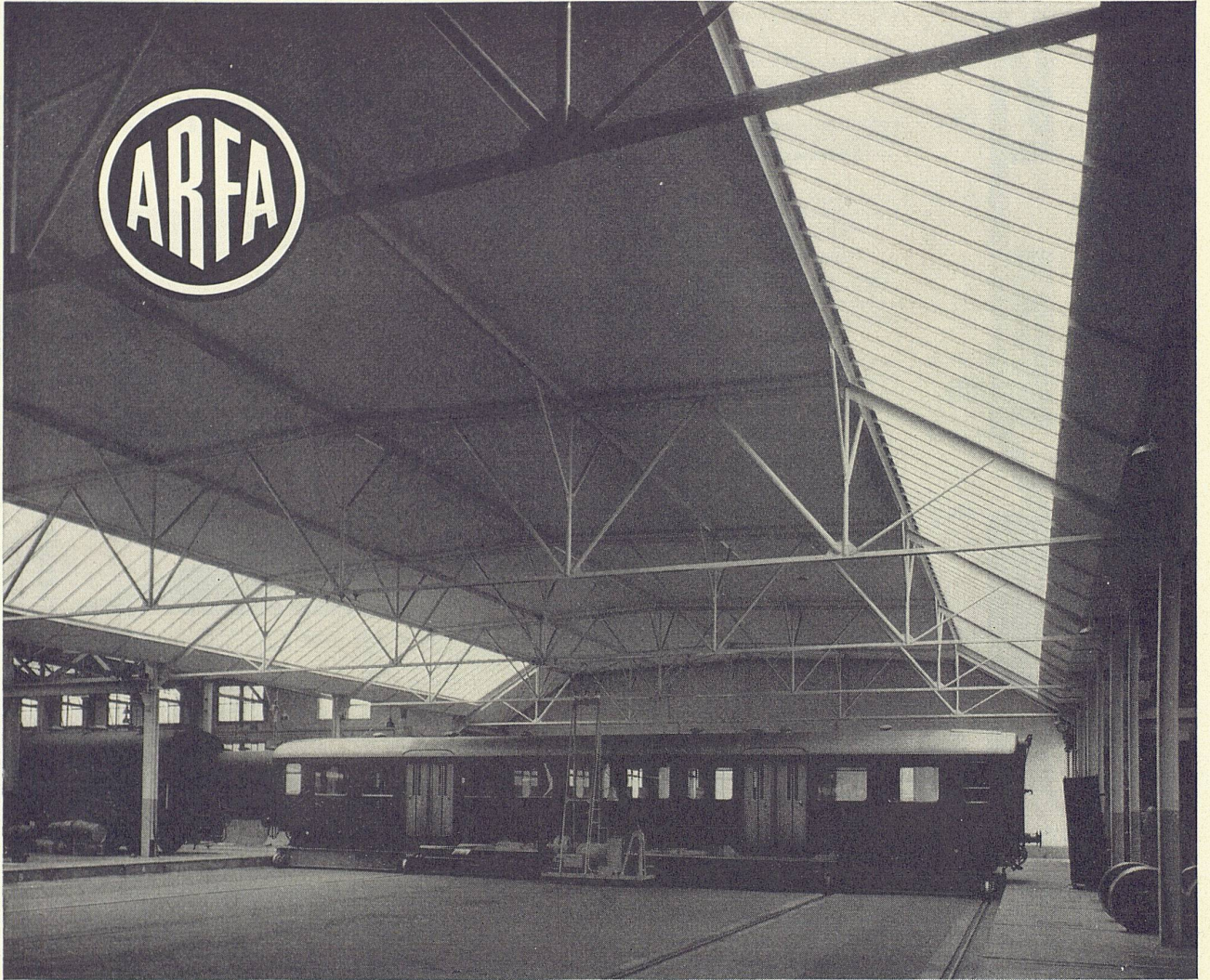
SBB Reparaturwerkstätte Olten, Binderkonstruktion ausgeführt mit ARFA Konstruktionsrohren durch Geilinger & Co., Winterthur
