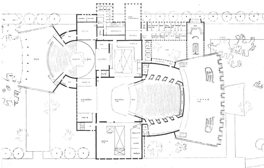
Hauptgeschoß ca. 1:1400. Axial verschobene Theatersäle mit getrennten Bühnen. Kleines Haus der Arenaform angenähert | Etage principal | Main floor
