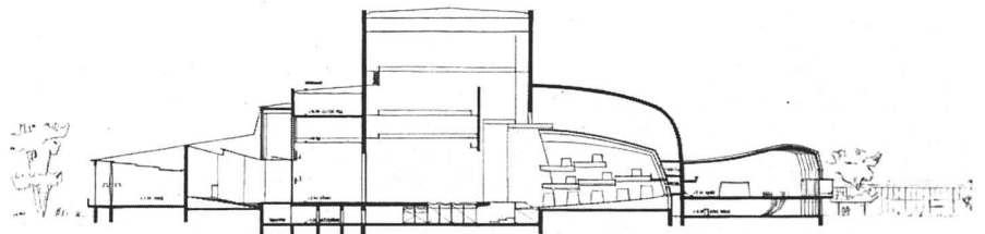
Längsschnitt ca. 1:1400 | Coupe longitudinale | Longitudinal cross-section
