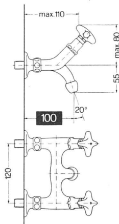
Überputz Hahnenndistanz 120 mm
