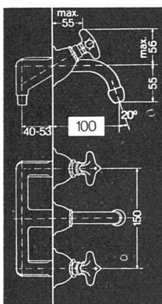
Unterputz Hahnenndistanz 150 mm
