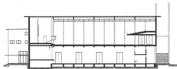
Längsschnitt 1:600
