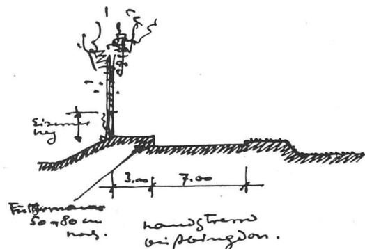
Landstrasse mit höhergelegtem Fussgängerweg bei Abingdon, zwischen Oxford und Bath. Ansicht und Schnitt 1:400
