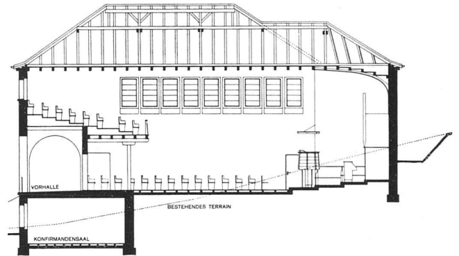
Längsschnitt 1 : 300
