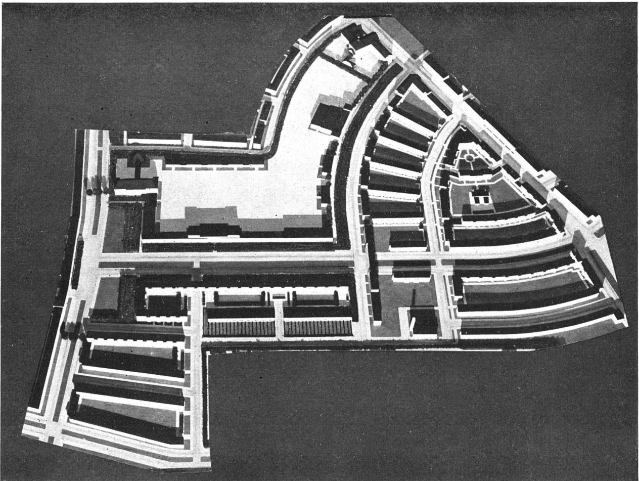
1200 WOHNUNGEN I. A. DER STADT BERLIN / IM BAU ARBEITSGEMEINSCHAFT AHRENDTS, BÜNING, PAULSEN / LEITUNG SALVISBERG
