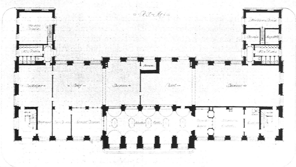
Bracher, Widmer und Daxelhofer, Architekten, Bern Post in Aarau. Grundriß Erdgeschoß, 1. und 2. Stock
