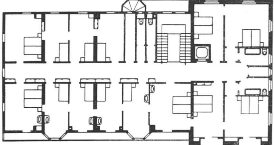
Maßstab 1 : 400 Grundriß II. Stock
