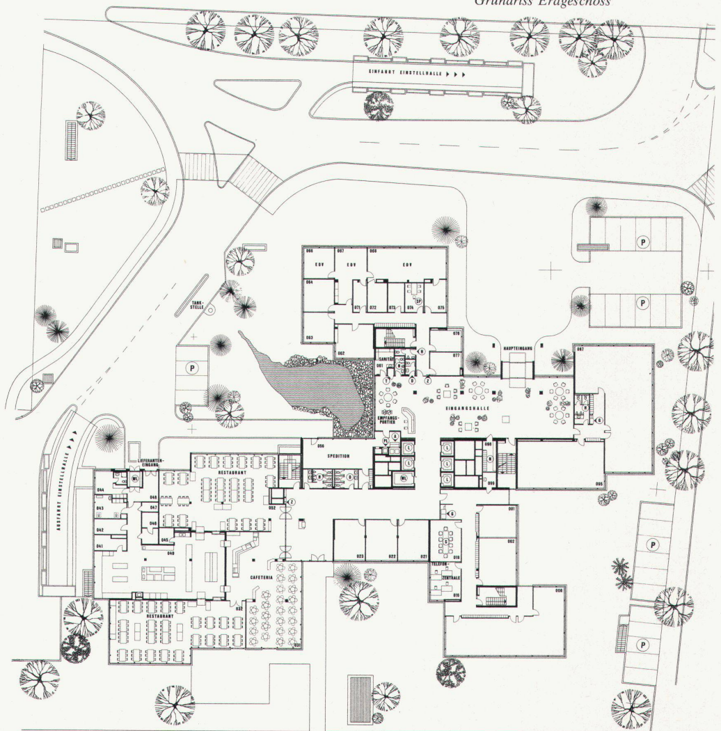
Grundriss Erdgeschoss
