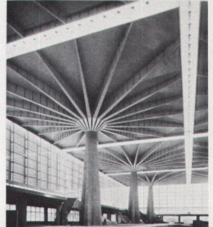
35 Palast der Arbeit in Turin, 1960–1961. Pier Luigi Nervi
