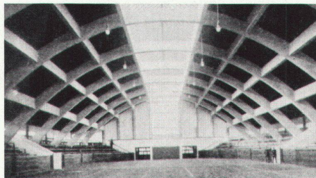
18 Sport- und Landwirtschaftshalle in Magdeburg, 1922. Bruno Taut mit Johannes Göderitz
