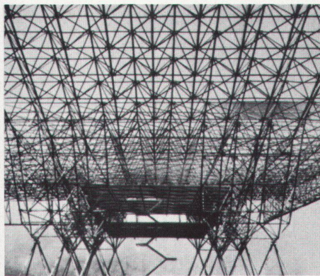
28 Konstruktionssystem für Hallenbauten, Projekt, 1950–1953. Konrad Wachsmann
