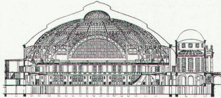
15 Festhalle in Frankfurt am Main, 1907–1909. Friedrich von Thiersch
