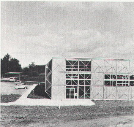
41 Lagerhalle in Weil am Rhein, BRD, 1971. Werner Blaser
