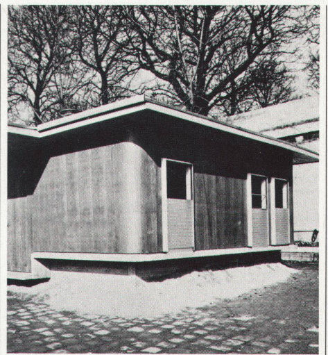
3 Prototyp des Hauses für Abbé Pierre, Paris, 1955–1956. Jean Prouvé
