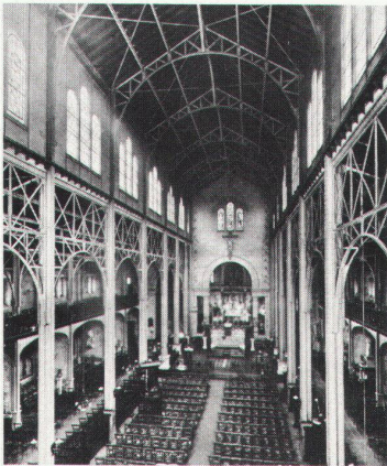
13 Kirche Notre-Dame du Travail, Paris, 1899. Astruc
