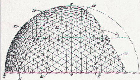
3 Geodätische Kuppel. R. Buckminster Fuller, 1954
