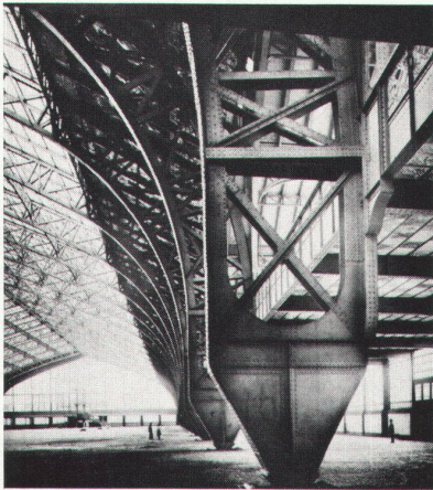
12 Maschinenhalle der Weltausstellung in Paris, 1889. Contamin und Dutert
