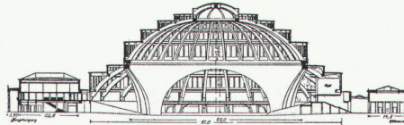
16 Jahrhunderthalle in Breslau, 1912–1913. Max Berg
