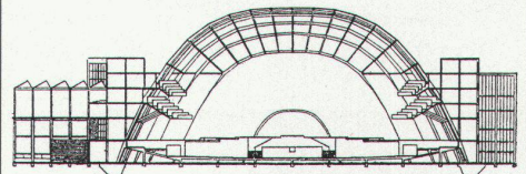
24 Projekt für das Völkerbundsgebäude in Genf, Saalbau, 1927. Hannes Meyer und Hans Wittwer
