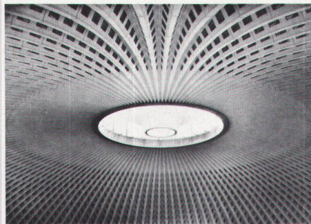
32 Palazzo dello Sport in Rom, 1958–1960. Pier Luigi Nervi
