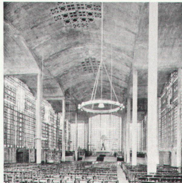
20 Kirche Notre-Dame in Raincy, Frankreich, 1922–1923. Auguste & Gustave Perret
