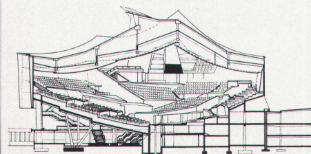
34 Konzerthaus der Berliner Philharmoniker, Berlin, 1956–1963. Hans Scharoun
