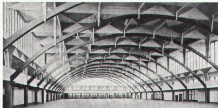
19 Messe-Halle in Breslau, 1922. Max Berg
