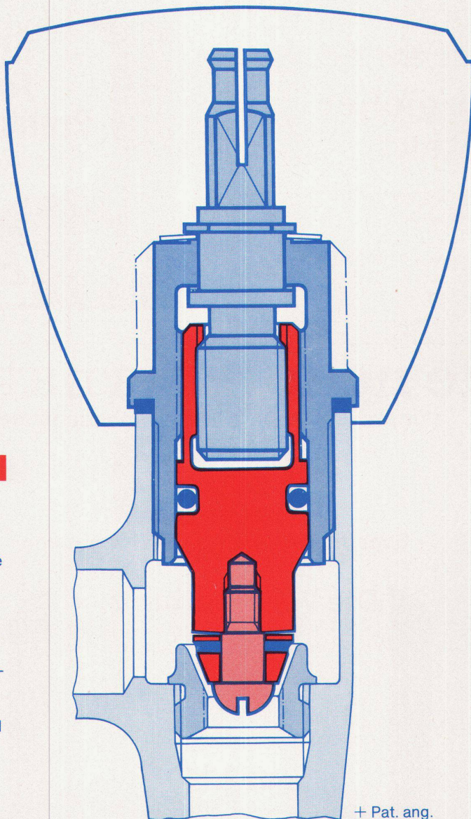
Stellung «open»
