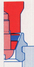
beim Schliessen Regulierkonus aufgesetzt, Dichtung nicht gepresst
