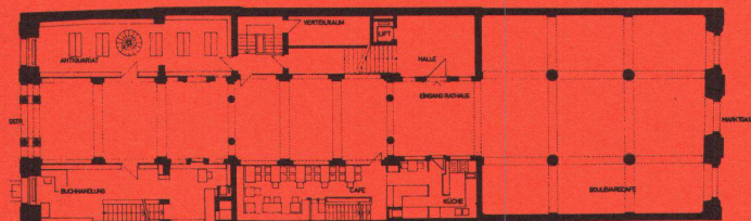
Grundriss Erdgeschoss mit Passage
