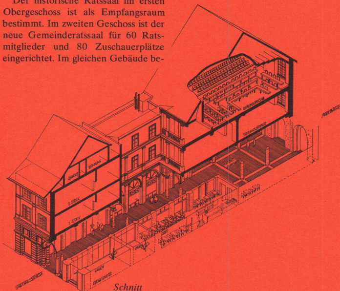
Schnitt
