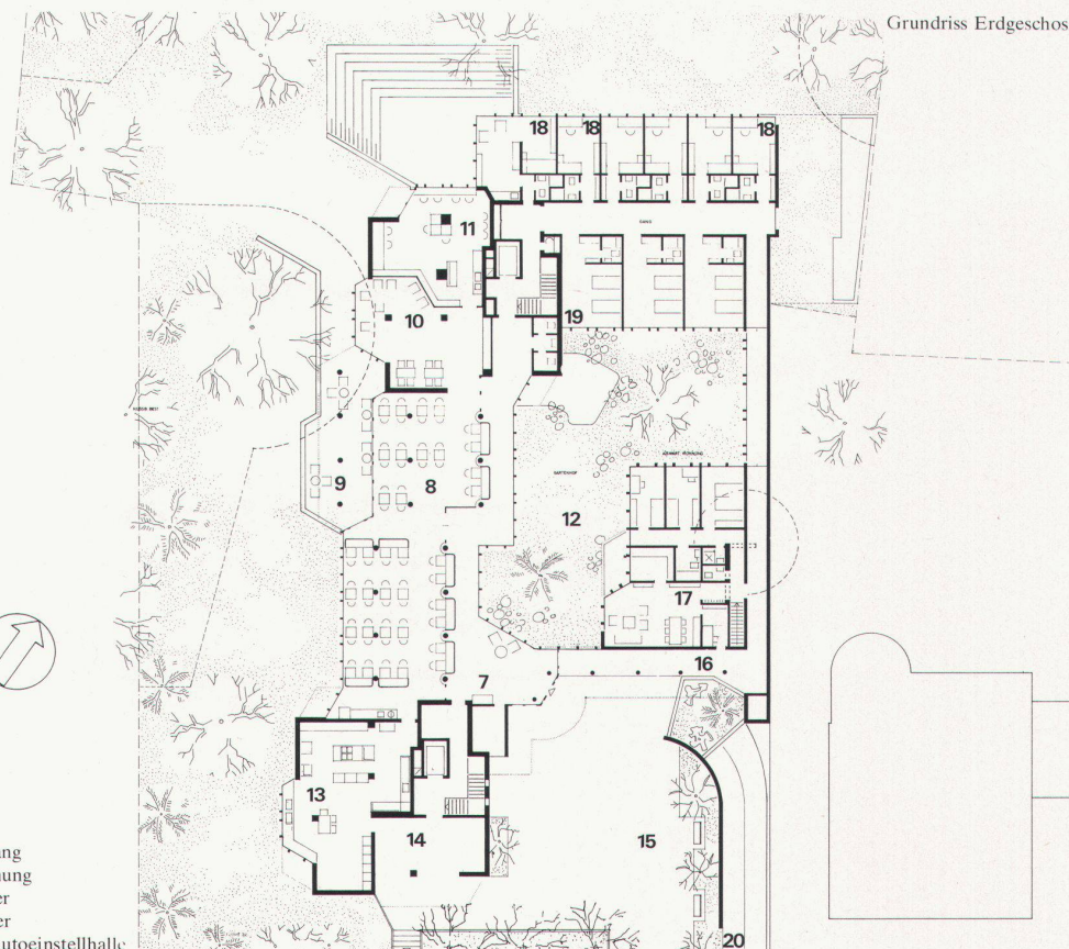
Grundriss Erdgeschoss
