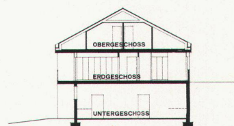
Schnitt durch Wohnhaus
