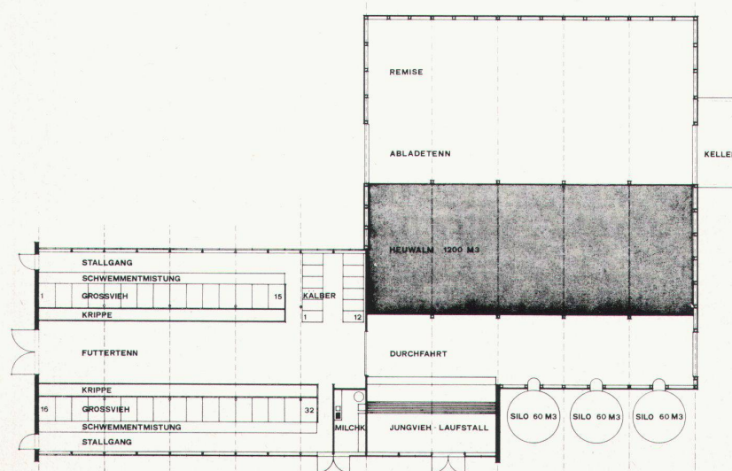
Grundriss Scheune
