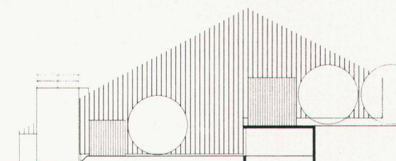
Nordostansicht Scheune
