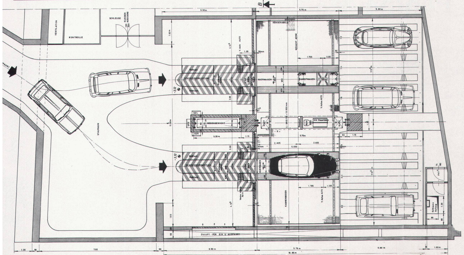
Grundriss: EINFABRTSGESCHOSS
