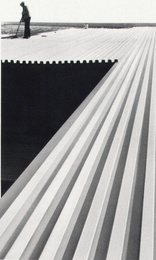
HOESCH TRAPEZPROFIL-DACH Warmdach-Aufbau: 1 HOESCH TRAPEZPROFIL 2 Bitumenveranstrich 3 Dämmung 4 Lachwiesbahn 5 Dachpappe V 11 6 Dachpappe V 13 blau beschiefert
