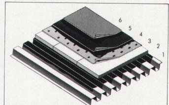
HOESCH TRAPEZPROFIL-DACH Warmdach-Aufbau: 1 HOESCH TRAPEZPROFIL 2 Bitumenveranstrich 3 Dämmung 4 Lachwiesbahn 5 Dachpappe V 11 6 Dachpappe V 13 blau beschiefert
