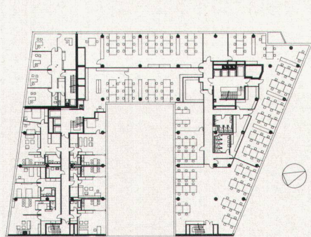
4. OBERGESCHOSS
