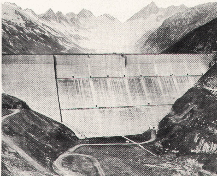
Oberaar-Staumauer
