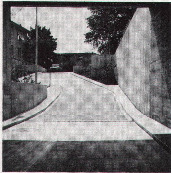
Ausführung von Duratex- Hartbeton und Novafalt Gussasphaltbelägen
