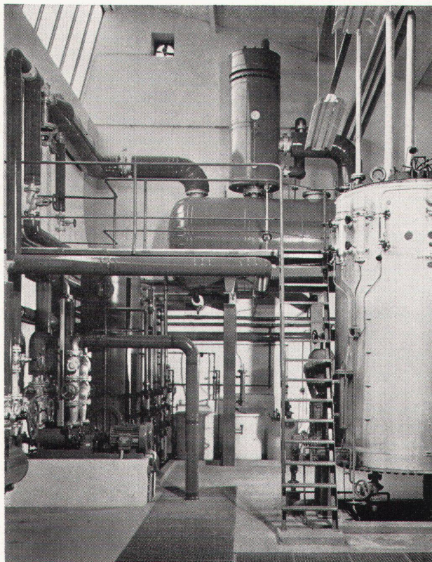
Aufbereitungs-Anlage für einen Mitteldruck-Kessel
