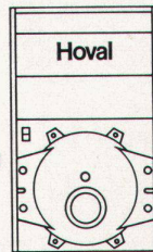
Hoval-Kessel Typ TG Gaskessel 14 000 bis 30 000 kcal/h
