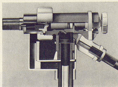
Neues GEBERIT-Schwimmerventil Modell 1970.
