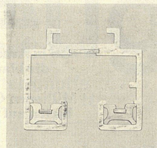
solide Leichtmetall-Stromschiene
