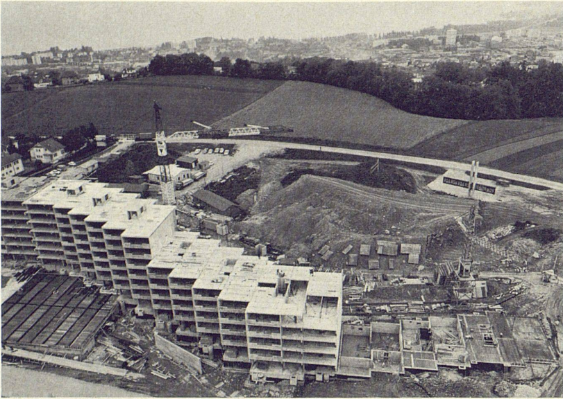
9, 10 Die Vorfabrikation kam mit insgesamt 54 Platten- typen aus; die Maße aller Teile sind gemäß der Modulordnung koordiniert 11 Südwestfassade
