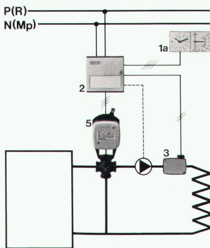
VILLAGYR RVK4(1) Stetige Raumtemperaturregelung
