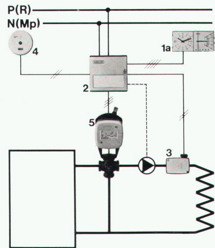
VILLAGYR RVK4(2) Stetige Raumtemperaturregelung, witterungskompensiert
