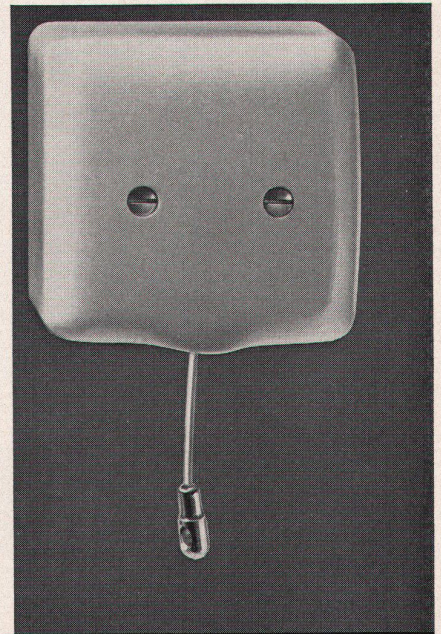
Zugschalter für Aufputz in trockenen Räumen ~10A, 250V
