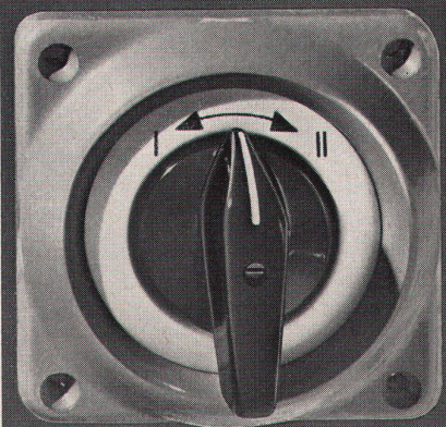
Schwenk- kontakt für den Einbau in Maschi- nen und Apparate ~6A, 500V
