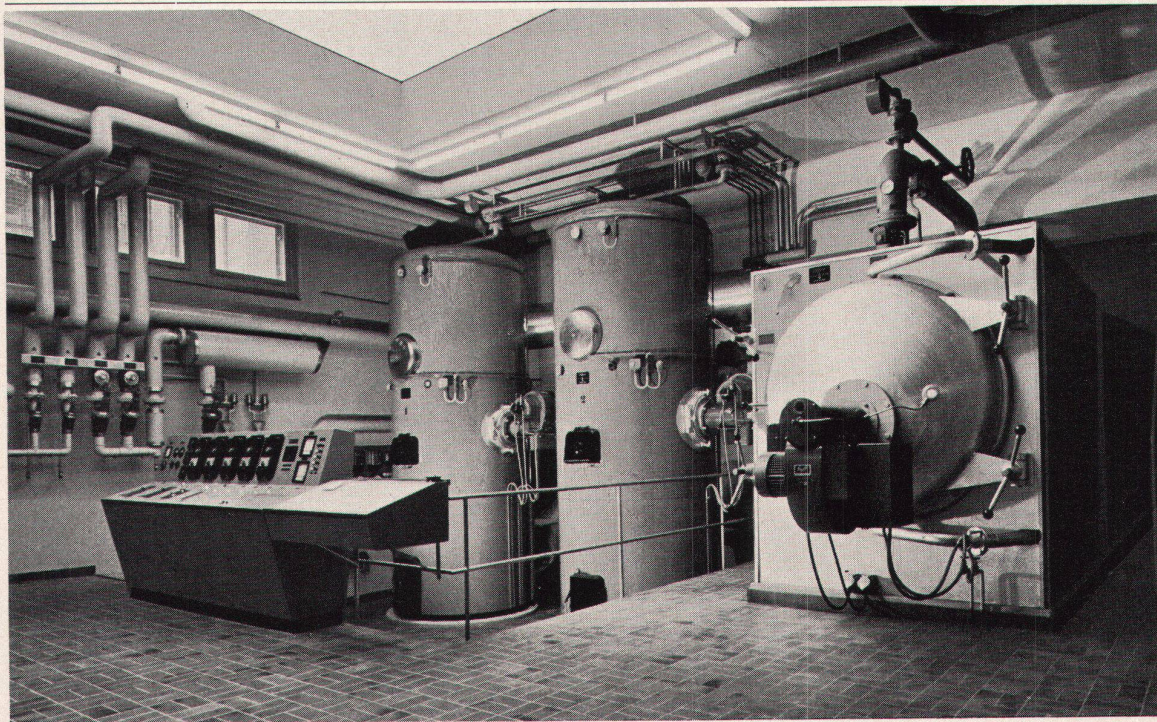
Ausgeführte Heizungs- und Lüftungsanlagen in Engelberg: Schulhaus Kloster
