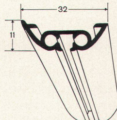
Silent Gliss Profil Spannfix 1041
