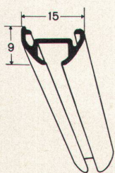
Silent Gliss Profil Spannfix 1060
