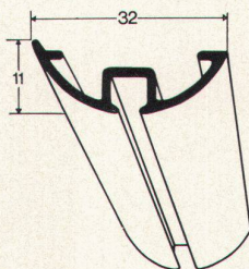
Silent Gliss Profil Spannfix 1048
