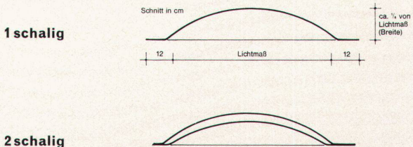
Form B zum Einbau auf Aufsatzkränze (mit oder ohne Lüftung)
