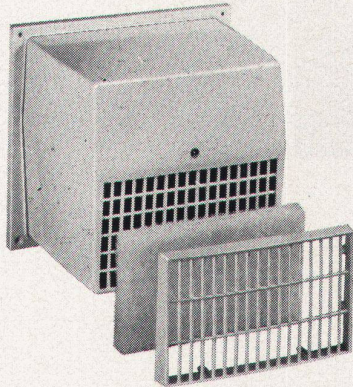
Schachtventilator Typ WKV 95
