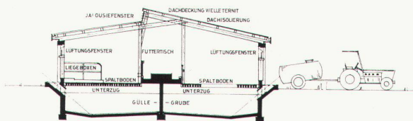
QUERSCHNITT GV-STALL
