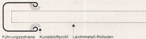
Führungsschiene Kunststoffprofil Leichtmetall-Rolladen
