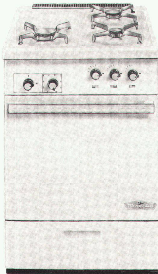
MENA-LUX/ARTHUR MARTIN 523 Einfaches Modell mit 3 Kochstellen. Normierte Dimensionen: 55/60/85
