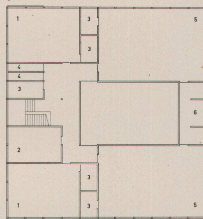
5 Block 4. Obergeschoß Annexe 4. Etage Block 4. Upper floor
