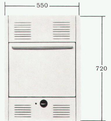
Dimensionen des Bono-Einbau-Backofens
