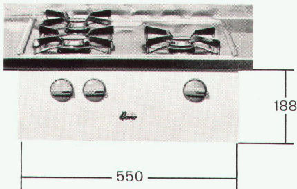
Dimensionen des Bono-Einbau-Kochtisches
