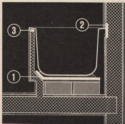
Wannenisolierung mit einer Korkplatte zwischen Boden und Untermuerung sowie Kork- oder Kunststoffstreifen unter und hinter dem Wannrand
