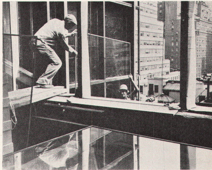
Die Glasscheibe wird eingesetzt. Weil die Kanten mit der Neoprene-Dichtung versehen sind, lässt sich das Glas leichter und sicherer handhaben.
