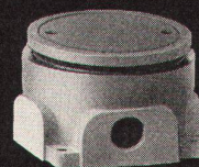
Bodendose mit Regulerring zur bodenbündigen Einstellung des Dosendeckels
