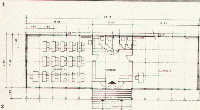
Vorfabrizierter, demontierbarer Schulpavillon in Thonex Architekt: Franz Amrhein, Genf
