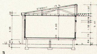
Vorfabrizierter, demontierbarer Schulpavillon in Thonex Architekt: Franz Amrhein, Genf
