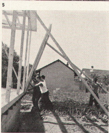
Vorfabrizierter, demontierbarer Schulpavillon in Thonex Architekt: Franz Amrhein, Genf
