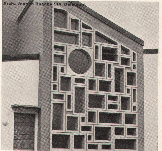
Betonsprossenfenster
