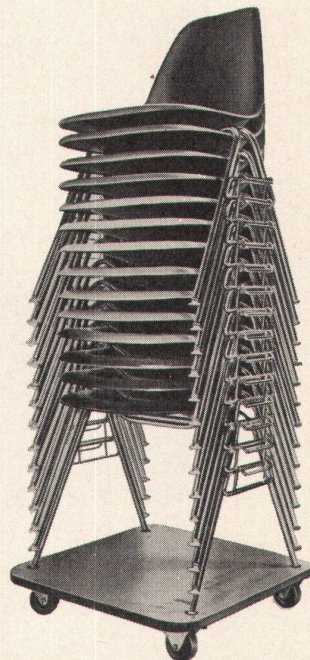
Dolly A Transportwagen für 15 DSS Dolly B Transportwagen für 30 DSS
