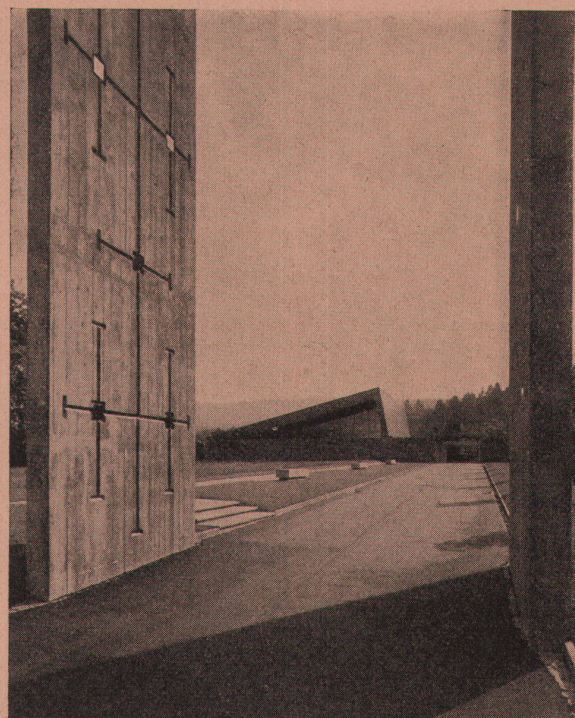
Ab dankungshalle und Krematorium Liebenfeld in Baden. Architekten: Edi und Ruth Lanners SIA und Res Wahlen SIA, Zürich
